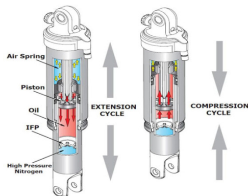
Gambar 2 : Penyerap Hentak Jenis Gas
