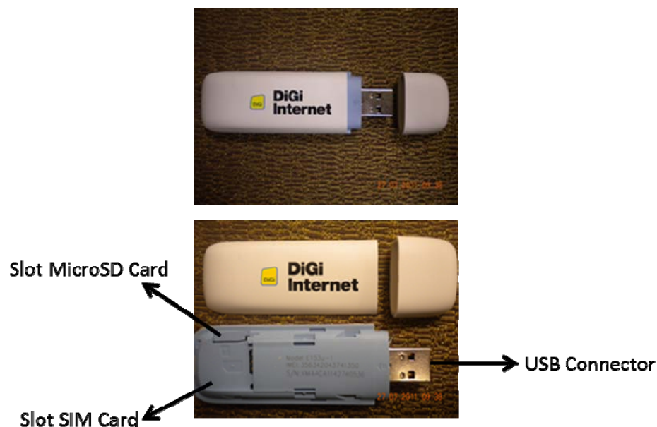
USB Modem Model : E153u-1 Brand : Huawei
